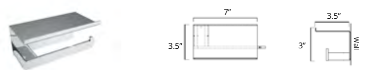
Toilet Paper Holder With Shelf Porte-papier toilette avec étagère
