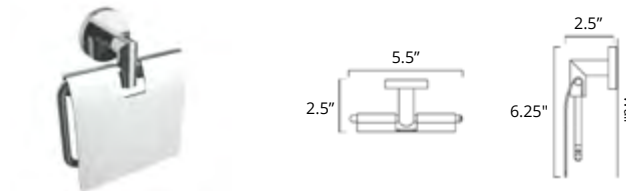
Pivot Toilet Paper Holder Porte-papier hygiénique pivotant
