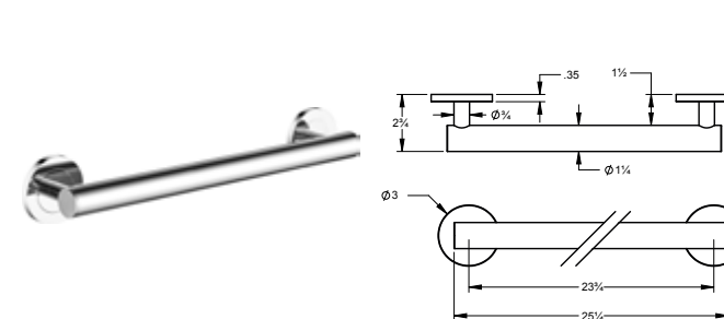
24" Lava Grab Bar Barre d'appui Lava 24"
