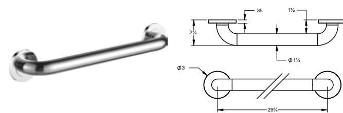
30" Round Grab Bar Barre d'appui ronde de 30"
