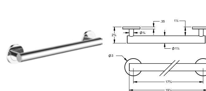
18" Lava Grab Bar Barre d'appui Lava 18"
