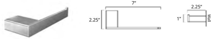
Toilet Paper Holder (RH) Porte-papier hygiénique (MD)
