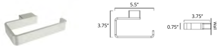
Toilet Paper Holder Porte-papier hygiénique
