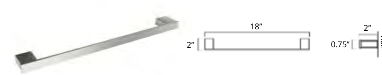
18" Towel Bar Porte-serviettes 18"
