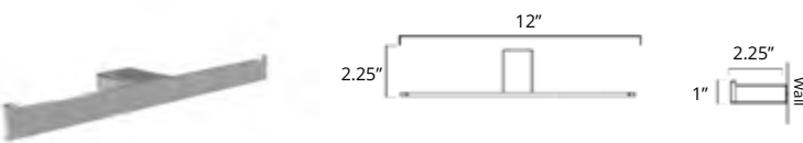
Double Toilet Paper Holder Double porte papier toilette
