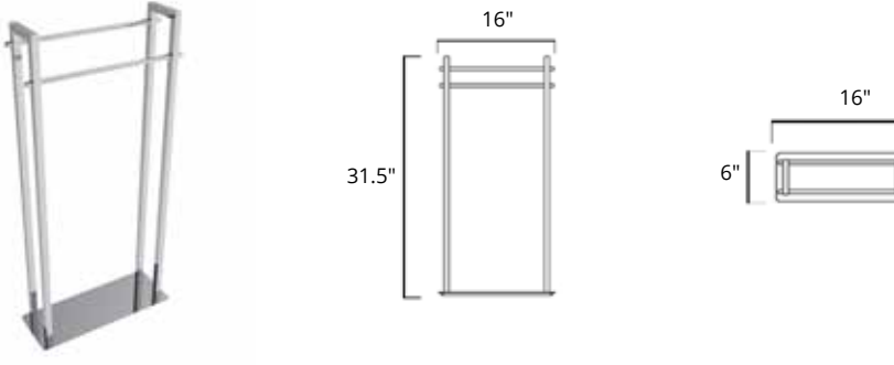
Square Freestanding Towel Stand Porte-serviettes sur pied carré
