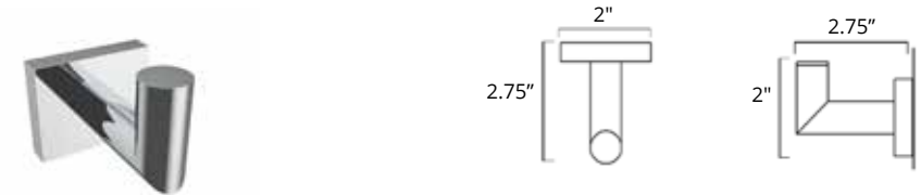
Towel Hook Crochet à serviette
