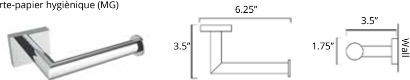
Toilet Paper Holder (LH) Porte-papier hygiénique (MG)
